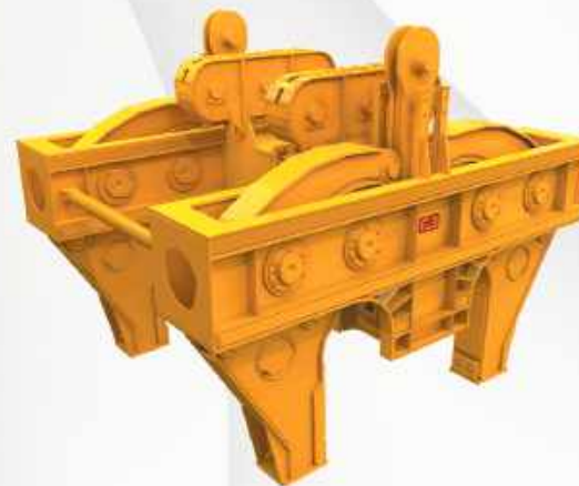
Клеши для слябов (г/п 115 т)
