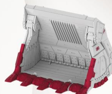
“Прямая лопата” для экскаватора
