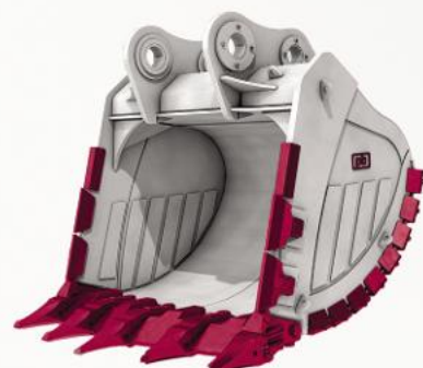
“Обратная лопата” для экскаватора
